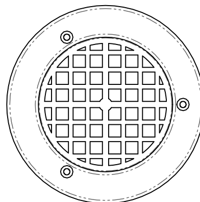
Innengitter 1019 Lochgröße 7x7 mm Lüftung 23 cm 3
