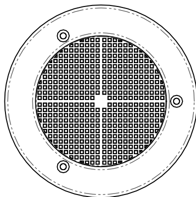
Innengitter 1006 Lochgröße 2x2 mm Lüftung 16 cm 3
