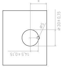
Schéma de perçage
