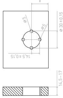
Schéma de perçage en option
